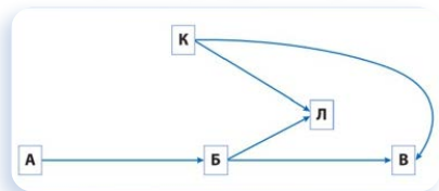
Рис. 2. Варіанти компонентів, що використовується при побудові орієнтованих ациклічних графів.
