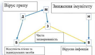
Рис. 1. Компоненти орієнтованих графів на прикладі визначення причинності розвитку вірусних інфекцій.
