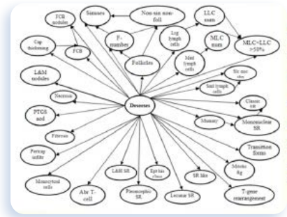
Рис. 3. Фрагмент байєсівської мережі побудованої на використанні ациклічних графів.
