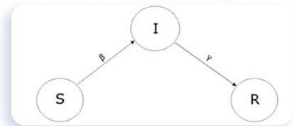
Рис. 4. Блок-схема показує перехід осіб-носіїв вірусу з одного стану в інший, чорні стрілки – швидкість переходу.
